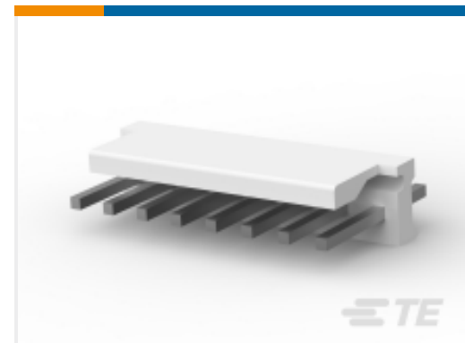
TE Part # 644752-8 08P MTA156 HDR ASSY SQ STR F/L
